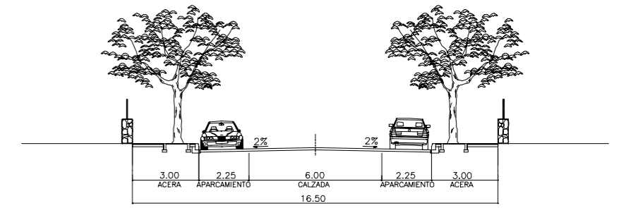
SECCIÓN TIPO 1
