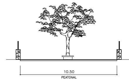
SECCIÓN TIPO 4
