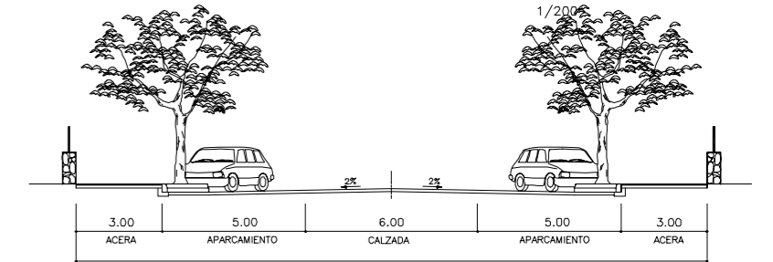
SECCIÓN TIPO 2
